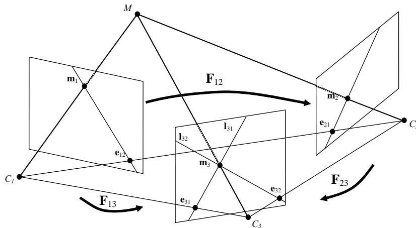
Abb. 10.1. Die erweiterte Epipolargeometrie für drei Ansichten
